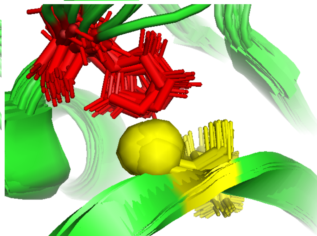
(d) 2KKZ L61-H86 (Ensemble)
