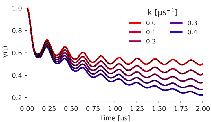
(b) Q-band ( \nu_T = 34.0 GHz)
